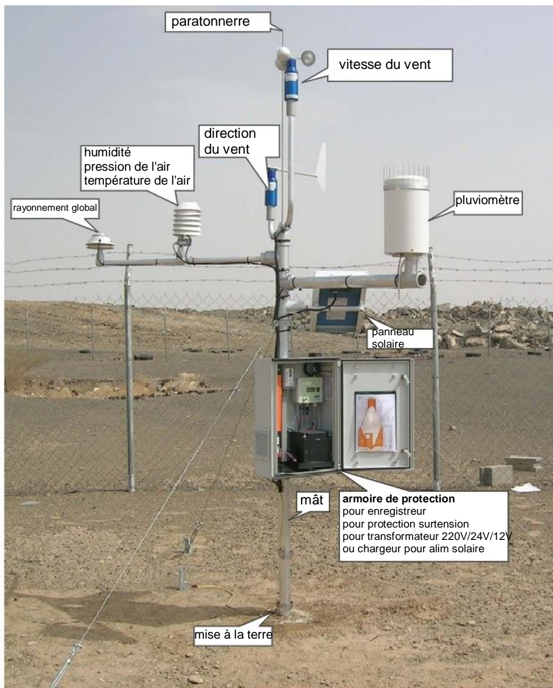
Exemple station météo complète (photo non contractuelle)
