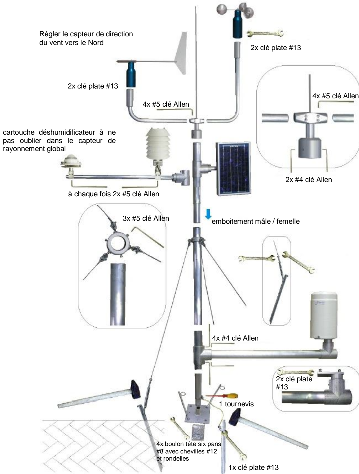
Schéma d'assemblage
