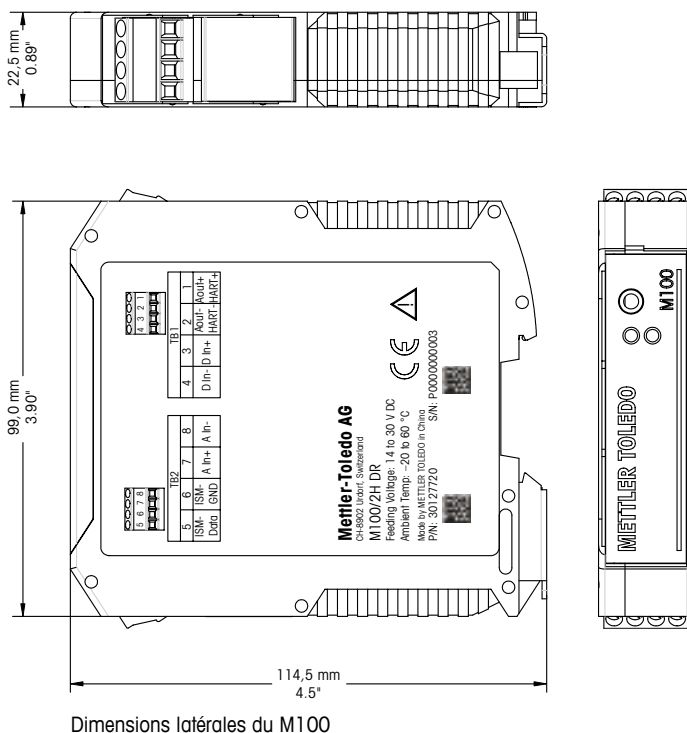
Dimensions latérales du M100
